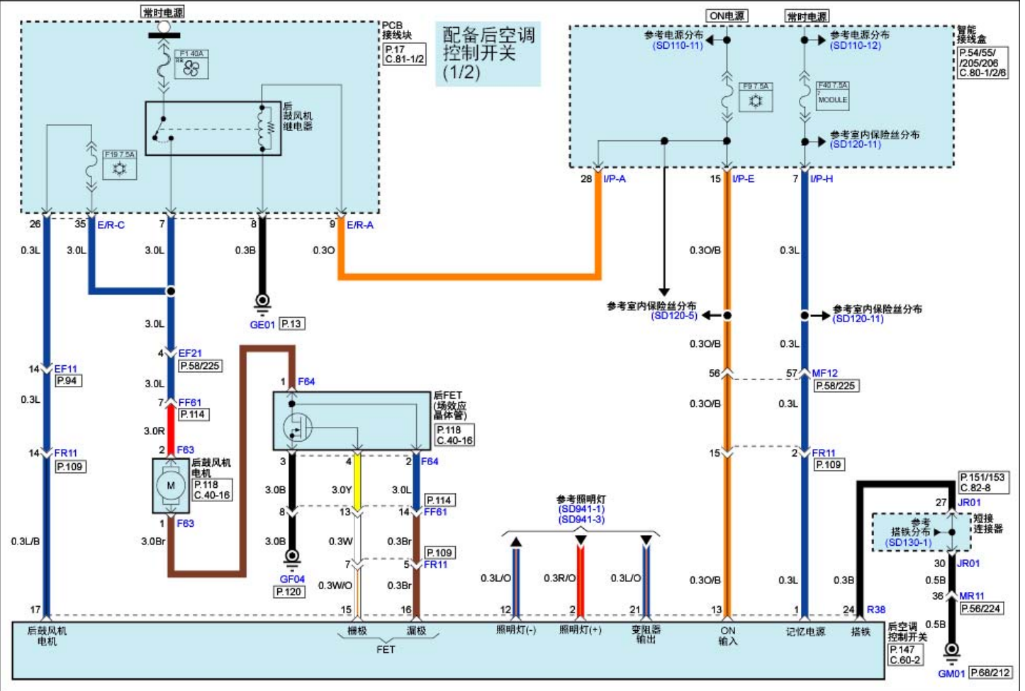
空调控制系统(手动)(6)
